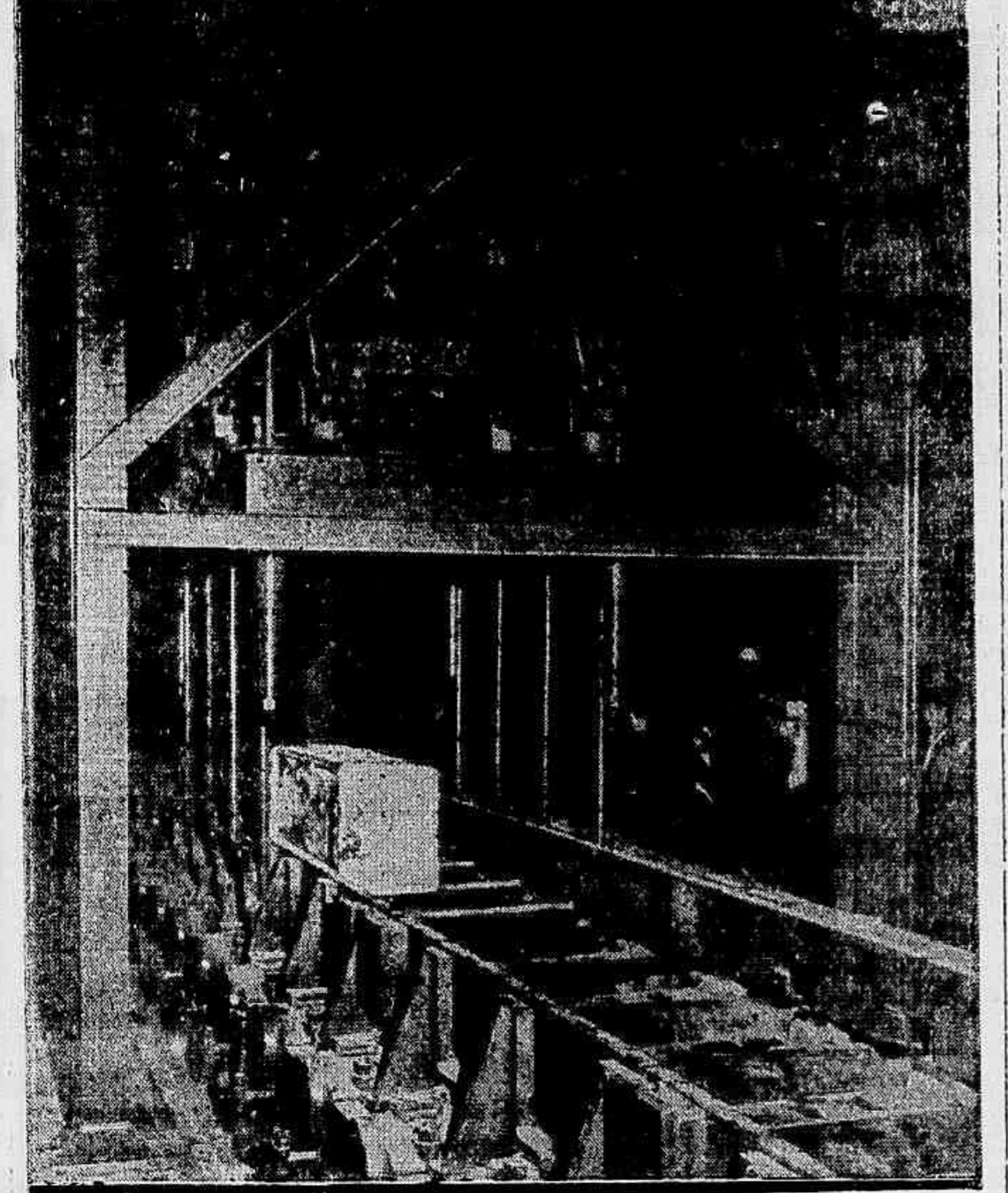
A gravura acima fixa o instante em que um lingote de aço é submetido ao laminador-desbastador. Daí para a frente, ele corre pela esteira volante sofrendo sucessivas pressões e moldagens, até se transformar no tipo de produto desejado. Este flagrante foi testado quando os representantes das classes produtoras de Minas Gerais visitaram a nossa grande usina siderúrgica.
