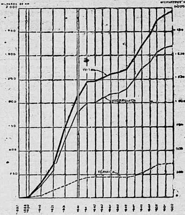
DESENVOLVIMENTO DA INDÚSTRIA DE ELETRICIDADE NO BRASIL CAPACIDADE DE GERAÇÃO INSTALADA
