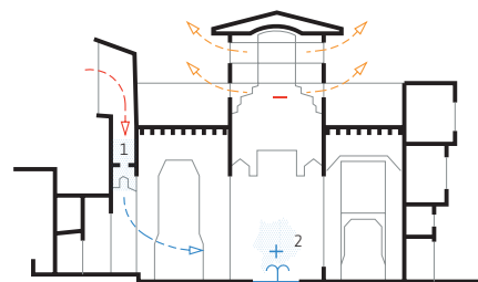
1 Recipientes de agua porosos 2 Vaporización de agua
