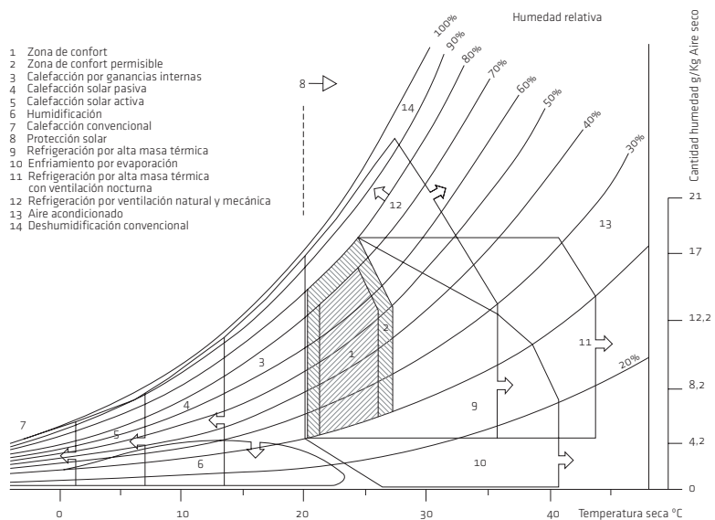
Fig.2.6. Diagrama de confort. Válido para 40° de latitud. Olgay(4) Fig. 2.7. Diagrama de confort. Givoni(4)
