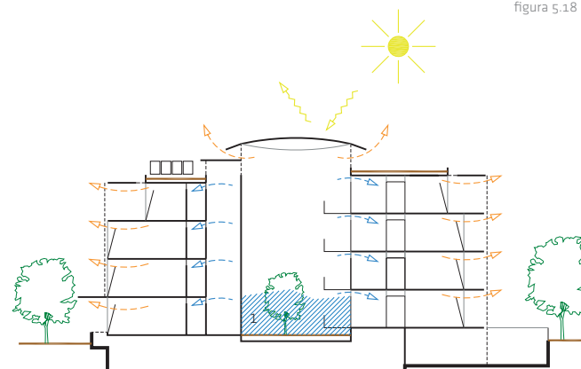
1 Piscina de aire frío
