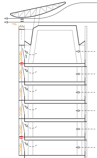
1 Doble carpintería. Hoja interior ventilada
