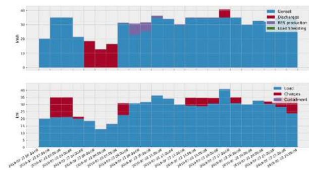
Figura 10. Potencia generada del caso PSDS utilizando un algoritmo MPC (controlador de optimización) el 23 de julio en Pojo Pata.
