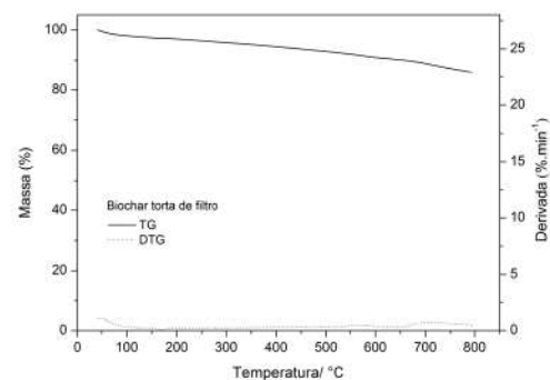
Figura 6. Curvas obtidas pela análise termogravimétrica da amostra de BTF.
