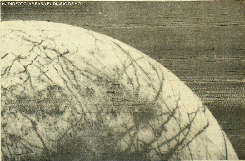
SATELITE DE JUPITER. — Pasadena, Estados Unidos, julio 11. Fotografía del satélite Europa, tomada por la nave Voyager 2, durante su aproximación a Júpiter, el 9 de julio. Europa que tiene el tamaño de la Luna de la Tierra, tiene probablemente 100 kilómetros de espesor.
