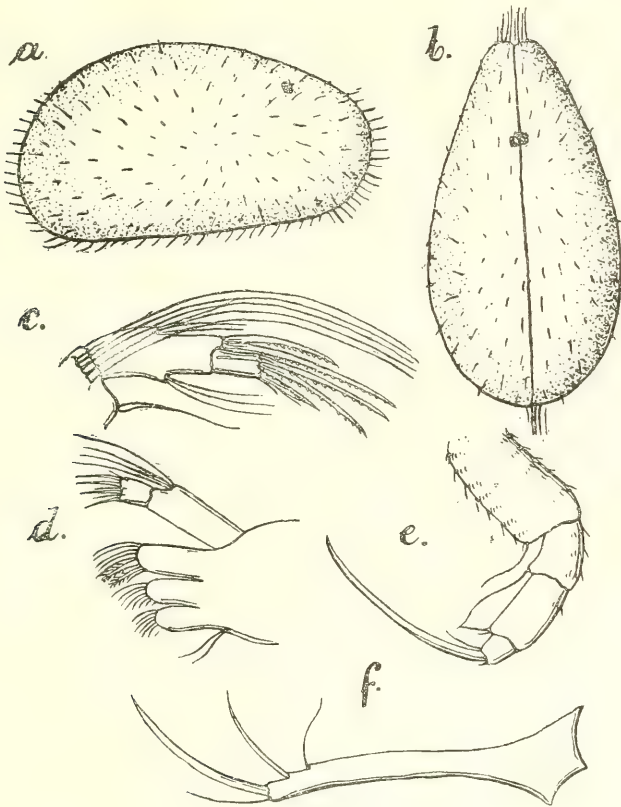
FIG. 4.— Eucypris tibetana , n. sp.
