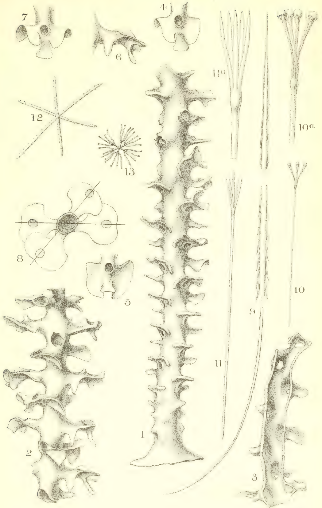
EURETE ANNANDALEI. n. sp.
