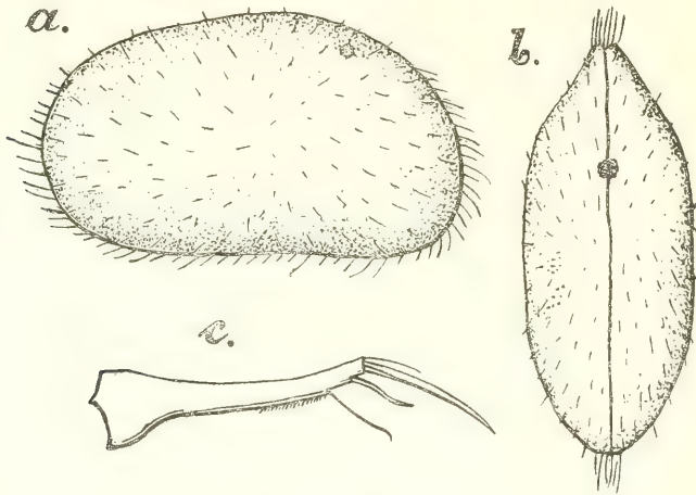
FIG. 5.— Eucypris minuta , n. sp.
