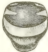
Megaspis errans , F.
